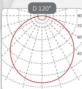
Схема распределения света для A3512PF-1SI, A3524PF-1SI, A3606PF-1SI, A3610PF-1SI, A3705PF-1SI, A3710PF-1SI
